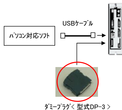
■ASEL/PSEL/SSEL用 USB接続パソコン対応ソフト 〈型式 IA-101-X-USB〉
