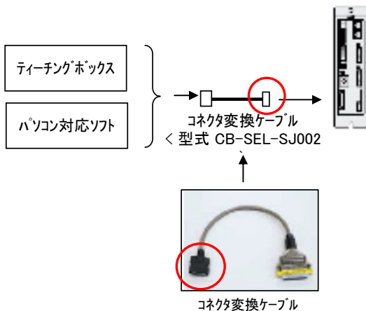
■ASEL/PSEL/SSEL用ティーチングボックス 〈型式 SEL-T(TD)-J〉 ■ASEL/PSEL/SSEL用パソコン対応ソフト 〈型式 IA-101-X-MW-J〉
