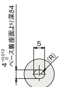
詳細図 P1 ベース長穴詳細
