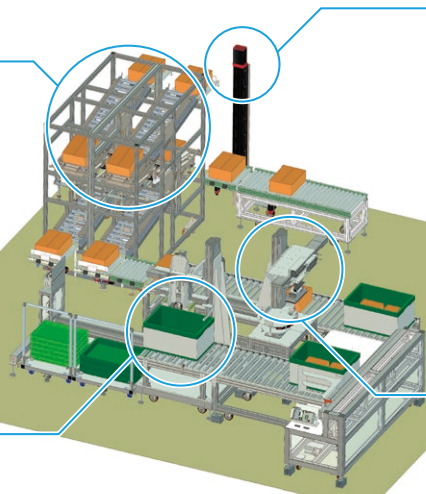
折りコン組立て+パッファユニット
