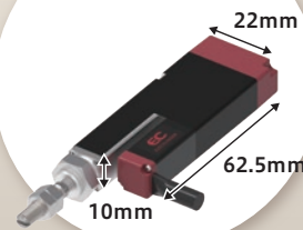
縦型グリッパー
