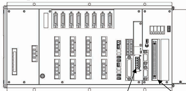
標準入力ポート No.0~191 標準出力ポート No.300~491 (DeviceNet ボード) 標準入力ポート No.192~239 標準出力ポート No.492~539 (I/O ボード)
