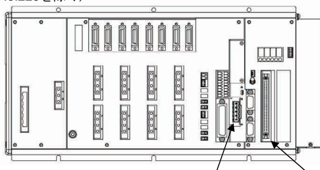
標準入力ポート No.0~15 使用しない(I/O ボード) 標準出力ポート No.300~315 (DeviceNet ボード)
