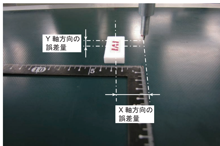
図 6-14 誤差量測定 01
