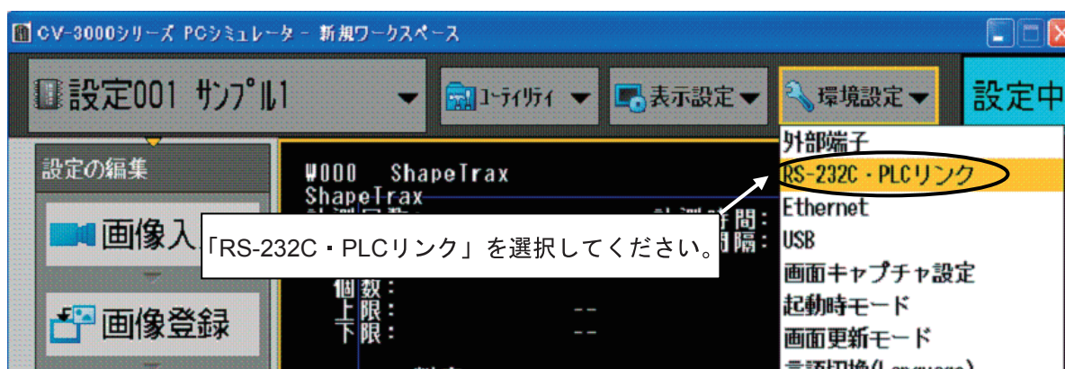
図 4-22 RS-232C・PLC リンク選択
