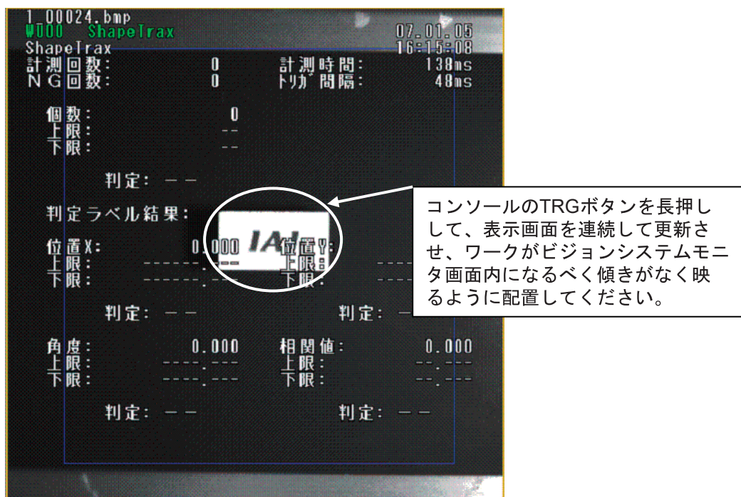
図 4-67 ワーク設置
