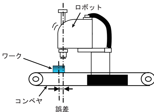
図 6-8 誤差確認
