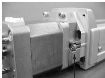
M3 × 18
