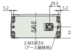
X軸背面 詳細
