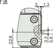
X軸側面Tスロット 詳細
