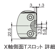
X軸側面Tスロット 詳細
