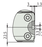
X軸側面Tスロット 詳細
