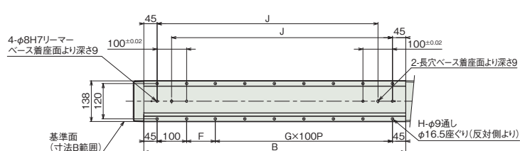
ベース取付寸法
