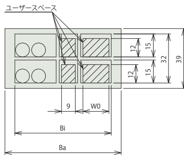
Y-Z間ケーブルキャリア断面図
