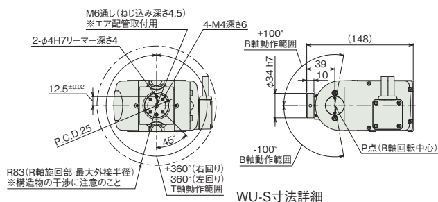
WU-S寸法詳細
