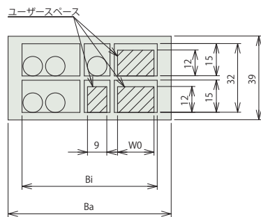
X-Y間ケーブルキャリア断面図
