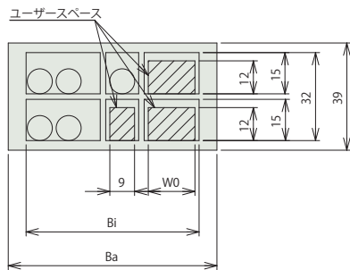
X-Z間ケーブルキャリア断面図
