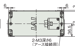
X軸背面 詳細
