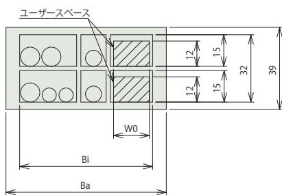
X-Y間ケーブルキャリア断面図
