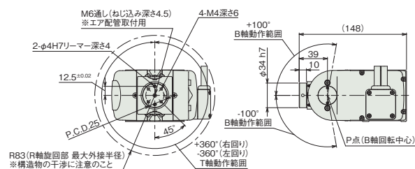
WU-S寸法詳細
