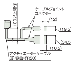
X軸ケーブル接続部
