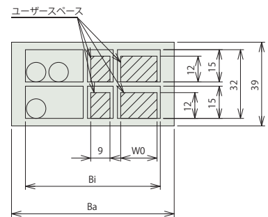
Z-R間ケーブルキャリア断面図
