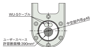
R軸中空部詳細
