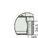
X軸ベース取付穴詳細
