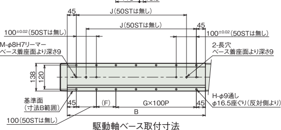
駆動軸ベース取付寸法
