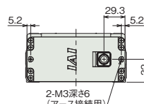
X軸背面 詳細
