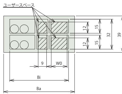
Z-Y間ケーブルキャリア断面図 Y-R間ケーブルキャリア断面図
