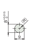
X軸ベース長穴詳細
