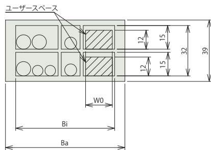
X-Z間ケーブルキャリア断面図
