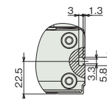
X軸側面Tスロット 詳細
