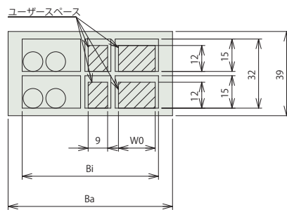
Z-Y間ケーブルキャリア断面図
