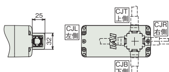
X軸ケーブル取出し方向(オプション)
