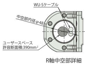
R軸中空部詳細
