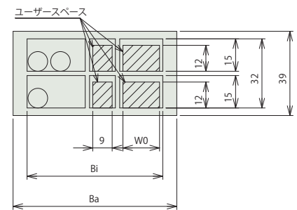
Y-R間ケーブルキャリア断面図
