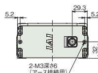
X軸背面 詳細
