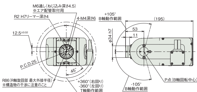
WU-M寸法詳細
