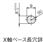
X軸ベース長穴詳細
