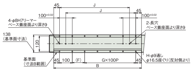
X軸ベース取付寸法
