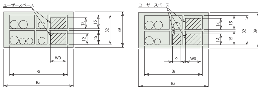
Y-Z間ケーブルキャリア断面図 Z-R間ケーブルキャリア断面図
