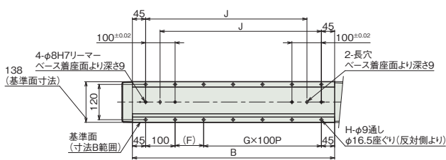
X軸ベース取付寸法
