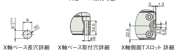
X軸ベース長穴詳細
