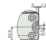
X軸側面Tスロット 詳細
