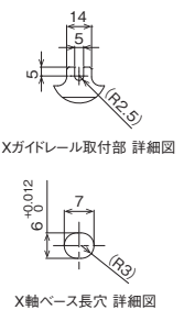
X軸ベース長穴 詳細図
