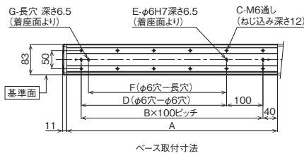
ベース取付寸法
