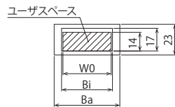
Z-Z間ケーブルキャリア断面図
