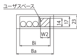
X-Y間ケーブルキャリア断面図
