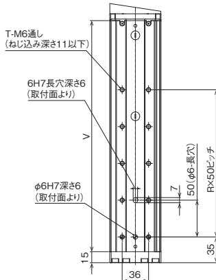
Y軸ベース長穴 詳細図
