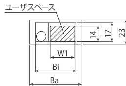
X-Y間、Y-Z間ケーブルキャリア断面図
