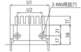
Y-Y間、Z-Z間ケーブルキャリア移動端詳細図 (CTL)
