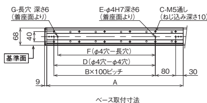
ベース取付寸法
