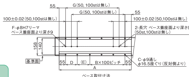
ベース取付寸法
