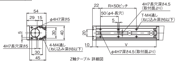
Z軸テーブル 詳細図
