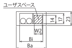
X-Y間ケーブルキャリア断面図
