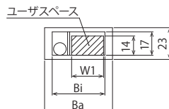
Y-Z間ケーブルキャリア断面図
