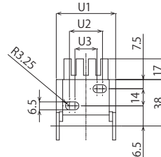
Y-Y間、Z-Z間ケーブルキャリア移動端詳細図 (CT,CTM)
