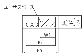
Y-Z間ケーブルキャリア断面図
