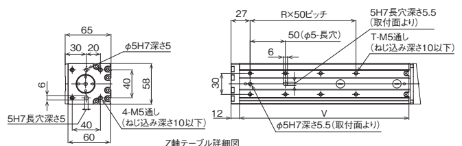
Z軸テーブル詳細図
