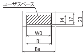
Y-Y間、Z-Z間ケーブルキャリア断面図
