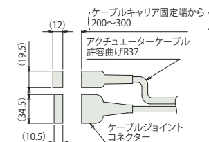
アクチュエーターケーブル接続部
