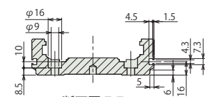
ベース取付け用深座ぐり穴詳細 Tスロット詳細
