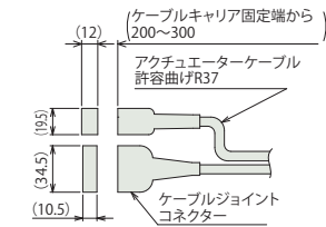
アクチュエーターケーブル接続部
