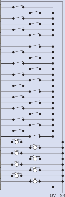
配線図
