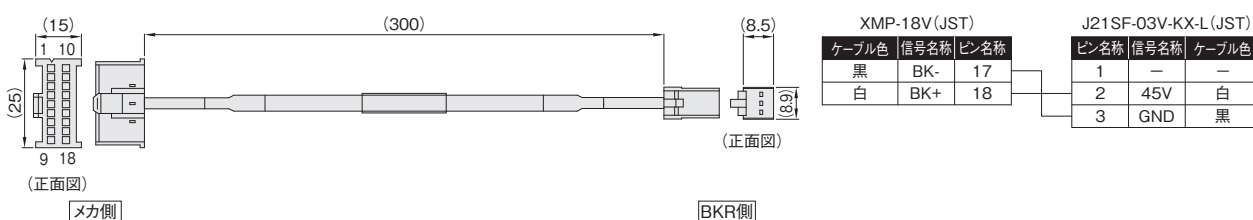
型式 CB-BK003-B31 ケーブル長0.3m
