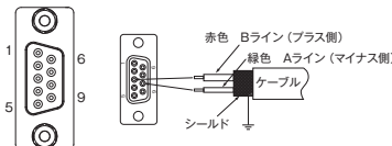
ネットワーク用コネクター
