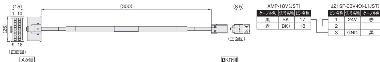
型式 CB-BK003-B12 ケーブル長0.3m
