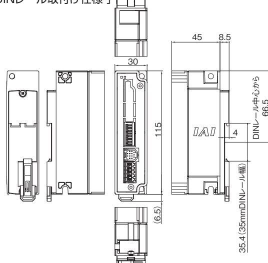
[DINレール取付け仕様]
