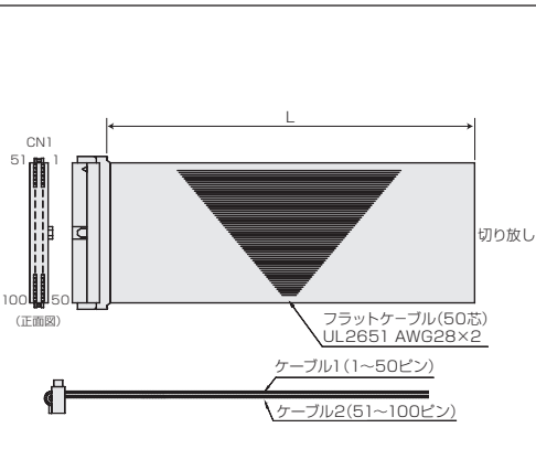
HIF6-100D1.27R(ヒロセ)
