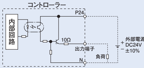
PNP仕様
