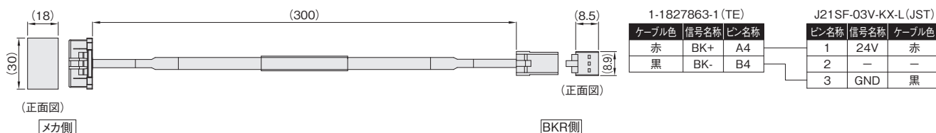
型式 CB-BK003-B12 ケーブル長0.3m
