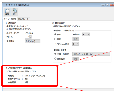
“ユーザーパラメーター編集”画面
