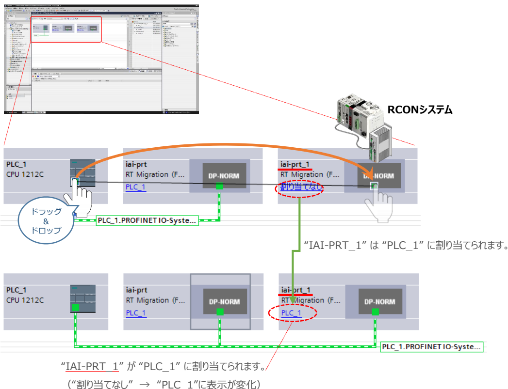
TIA Portal メイン画面
