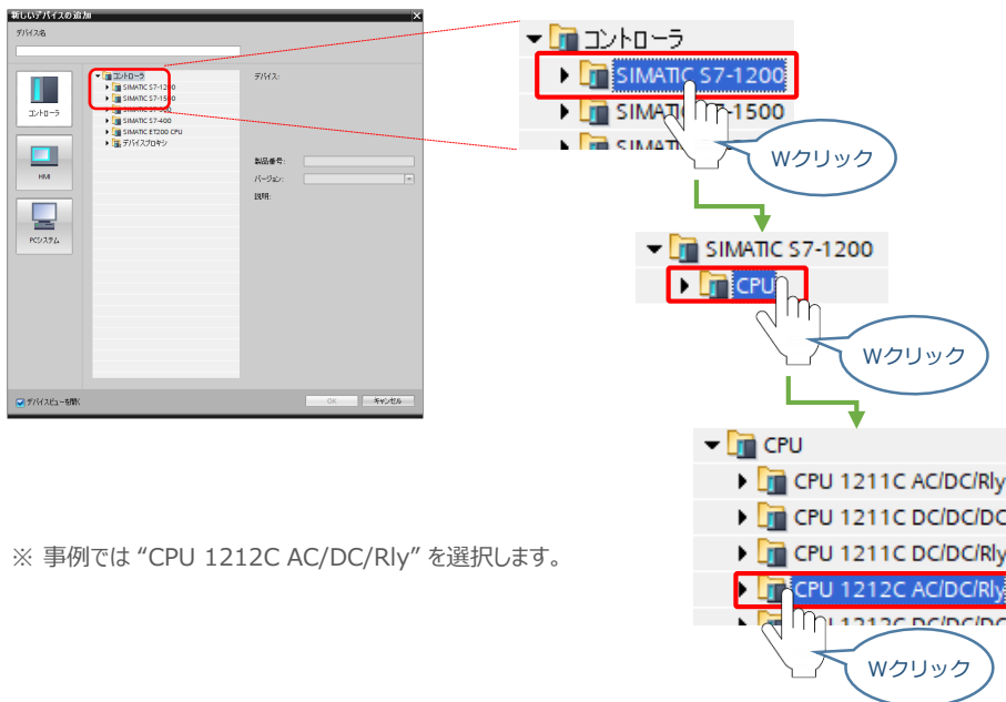
新しいデバイスの追加 画面
