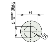
詳細図 Q フロントプレート長穴詳細
