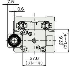
ケーブル取出し方向変更(左側) (型式CJL)
