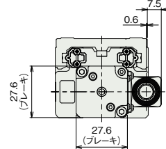
Rケーブル取出し方向変更(右側) (型式CJR)
