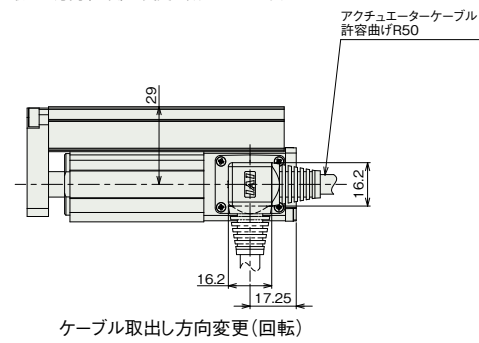
ケーブル取出し方向変更(回転)
