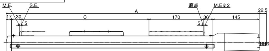
RCS3-SS8C-150
