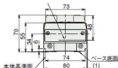
RCS3-SS8C-150
