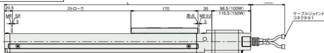
RCS3-SS8C-150
